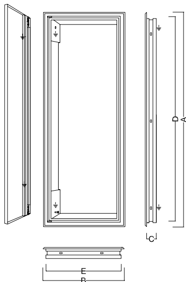
RAMA ROZDZIELNICI PODTYNKOWEJ
